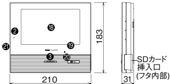
WJ-DA
