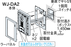
WJ-DA2
